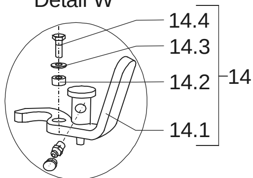
Einzelheit W Detail W
