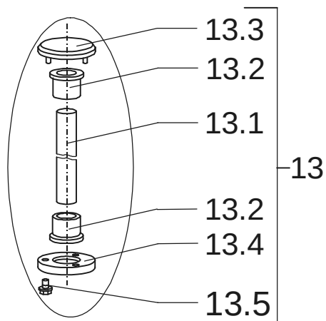
Einzelheit Y Detail Y
